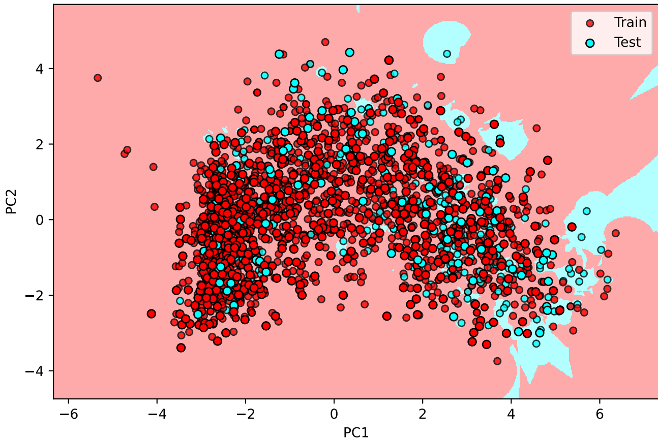
Frontera KNN en plano PCA (k=5, weights='distance')
